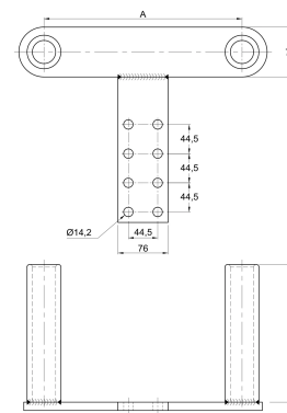
PLANO 2D · DIMENSIONES (MM)
