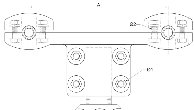
PLANO 2D · DIMENSIONES (MM)
