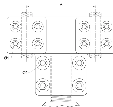
PLANO 2D · DIMENSIONES (MM)
