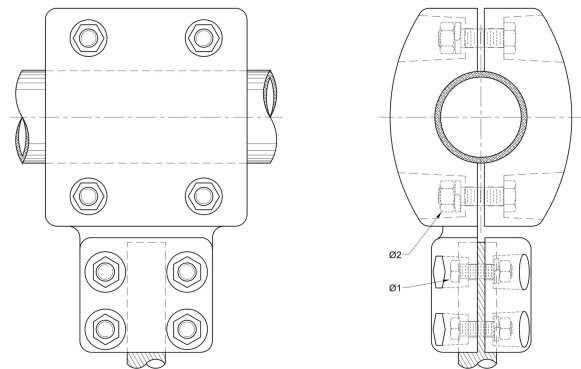
PLANO 2D · DIMENSIONES (MM)
