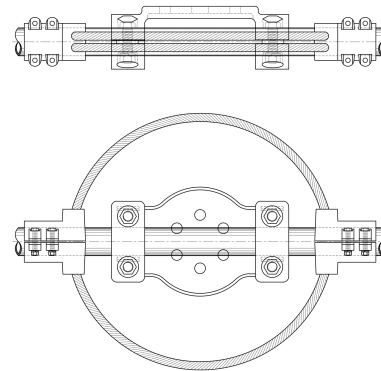
PLANO 2D · DIMENSIONES (MM)
