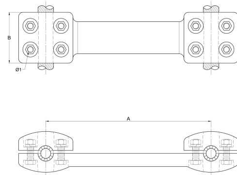
PLANO 2D · DIMENSIONES (MM)
