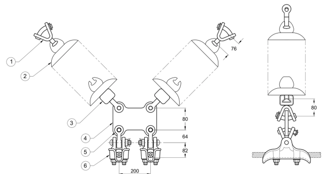
PLANO 2D · DIMENSIONES (MM)
