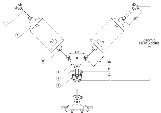
PLANO 2D · DIMENSIONES (MM)
