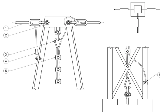
PLANO 2D · DIMENSIONES (MM)
